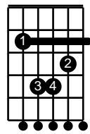
Bm
