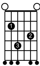
Em7(9)/B
