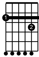
F#m7(#5)
