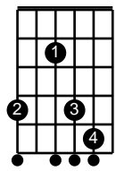
E/G#
