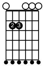
Em
