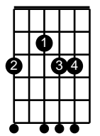
Gm6
