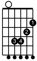
Bm/A
